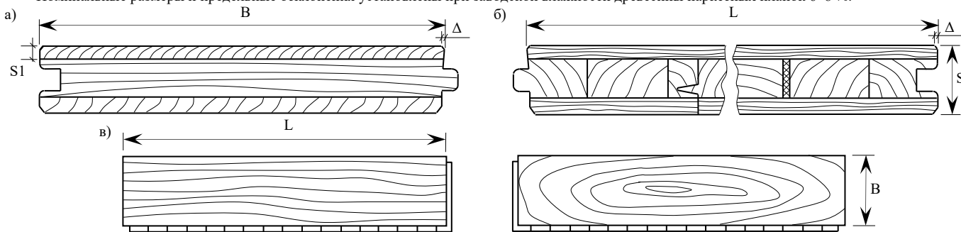
Рисунок 1: а) поперечный профиль, соединение T&G (паз-гребень); б) продольный профиль, соединение T&G (паз-гребень); в) внешний вид паркета.
